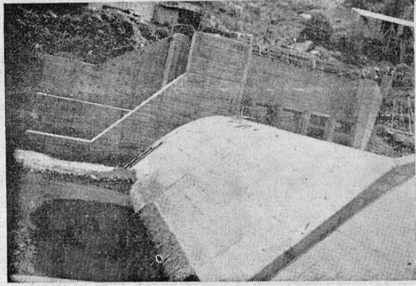
Aquí puede verse la enorme presa totalmente terminada, después de varios meses de intensa y vigorosa labor; el río tuvo que ser desviado para poder llevar a cabo su construcción. Lo que ahora se ve cubierto de piedras, será donde el agua forme la presa.
